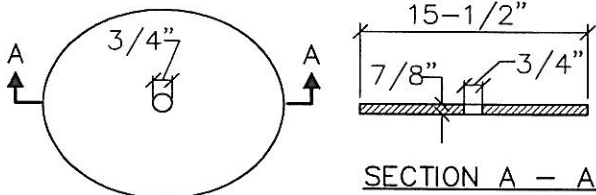
CLEANOUT LID
